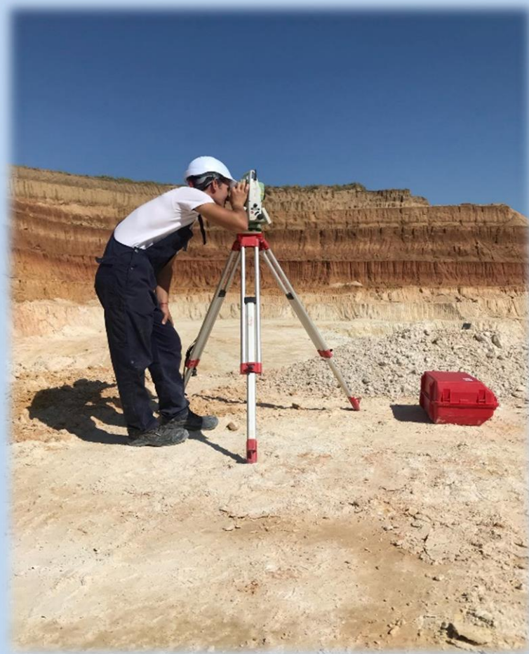
Извършване на оперативна снимка в рудник Есениците, Ветово
